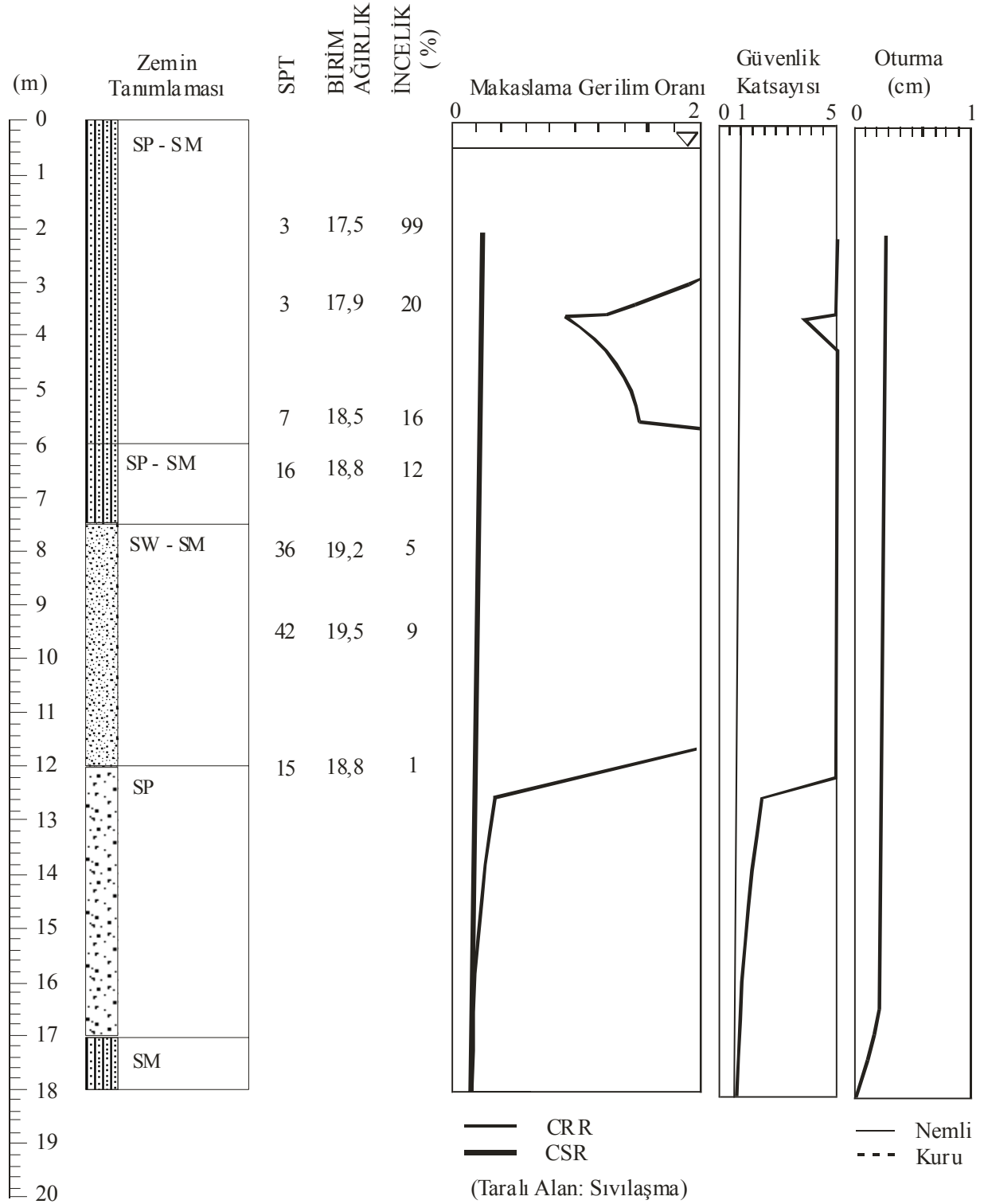
Şekil 11b: SK 37 kuyusu verilerine göre, 50 metrelik bir yapı yükü altındaki, sıvılaşma analiz Figure 11b: Liquefaction analysis under 50m structural load for data from borehole SK37
